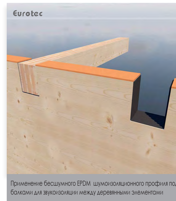
Бесшумный EPDM - шумоизоляционный профиль для разделения материалов и шумоизоляции
