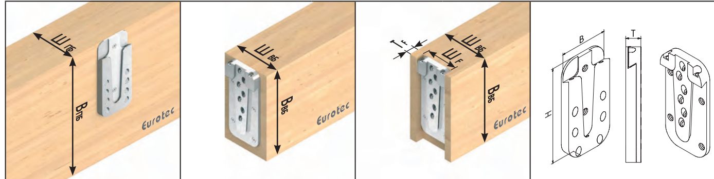
Условные обозначения: пролетная балка, второстепенная балка открытй монтаж, второстепенная балка потайной монтаж, размеры навесок
