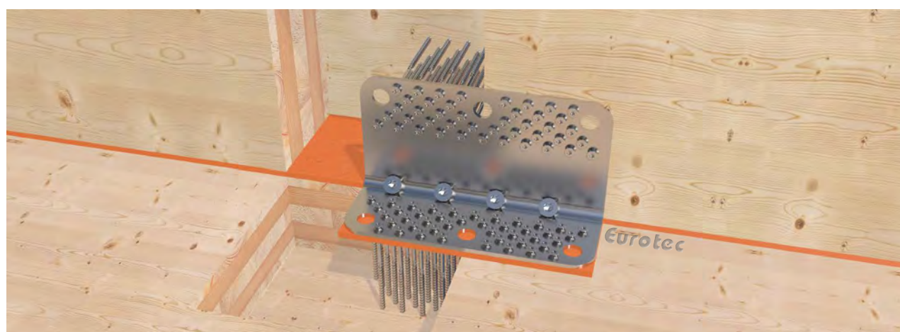
Уголок CLT в креплении стены к деревянному полу верхнего этажа.
