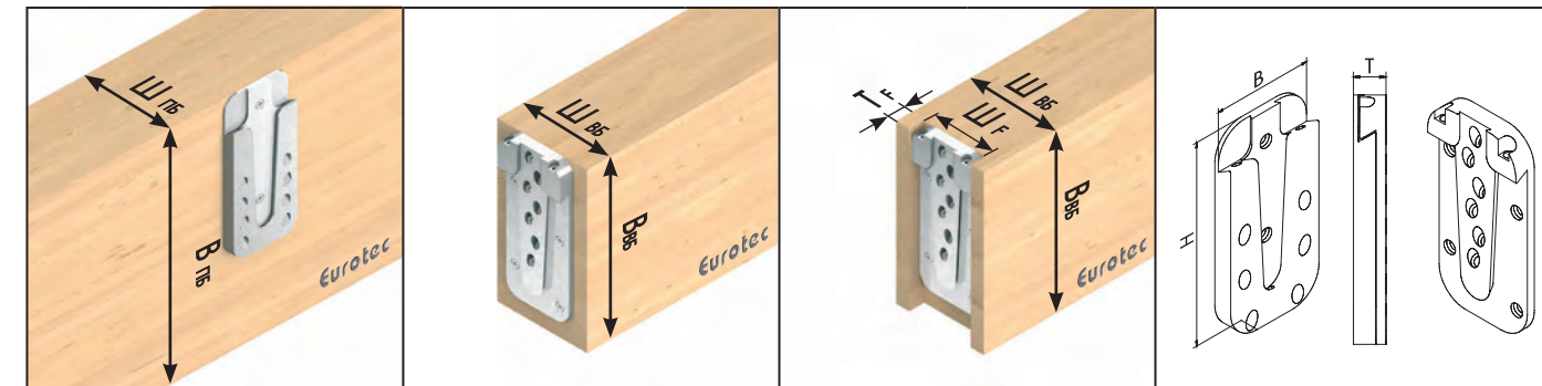
Условные обозначения: пролетная балка, второстепенная балка открытый монтаж, второстепенная балка потайной монтаж, размеры навесок
