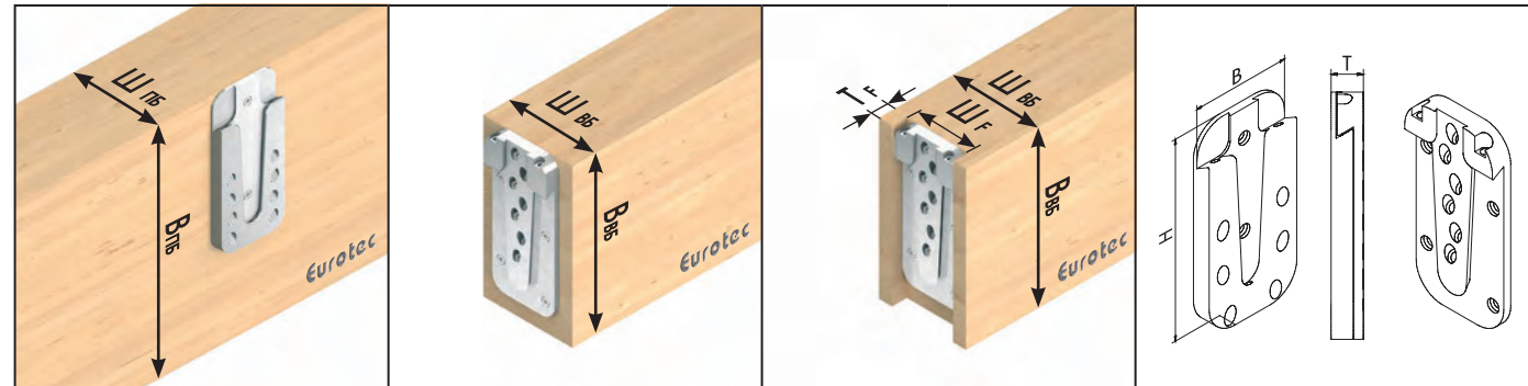
Условные обозначения: пролетная балка, второстепенная балка открытый монтаж, второстепенная балка потайной монтаж, размеры навесок
