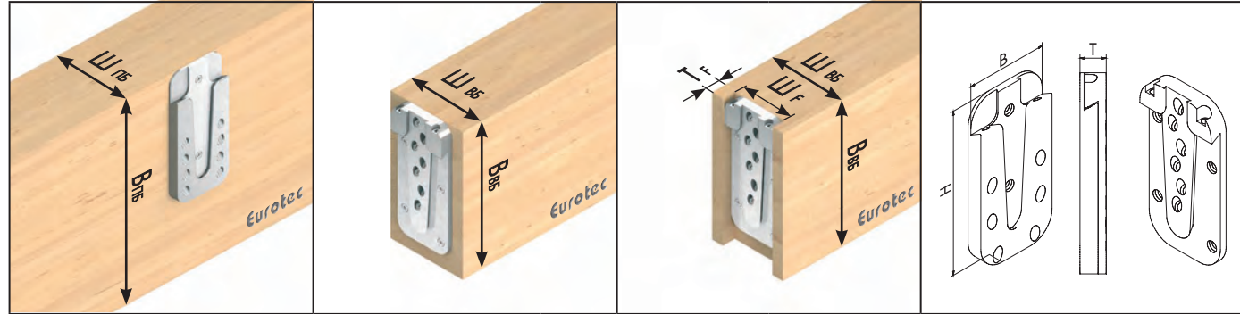
Условные обозначения: пролетная балка, второстепенная балка открытй монтаж, второстепенная балка потайной монтаж, размеры навесок
