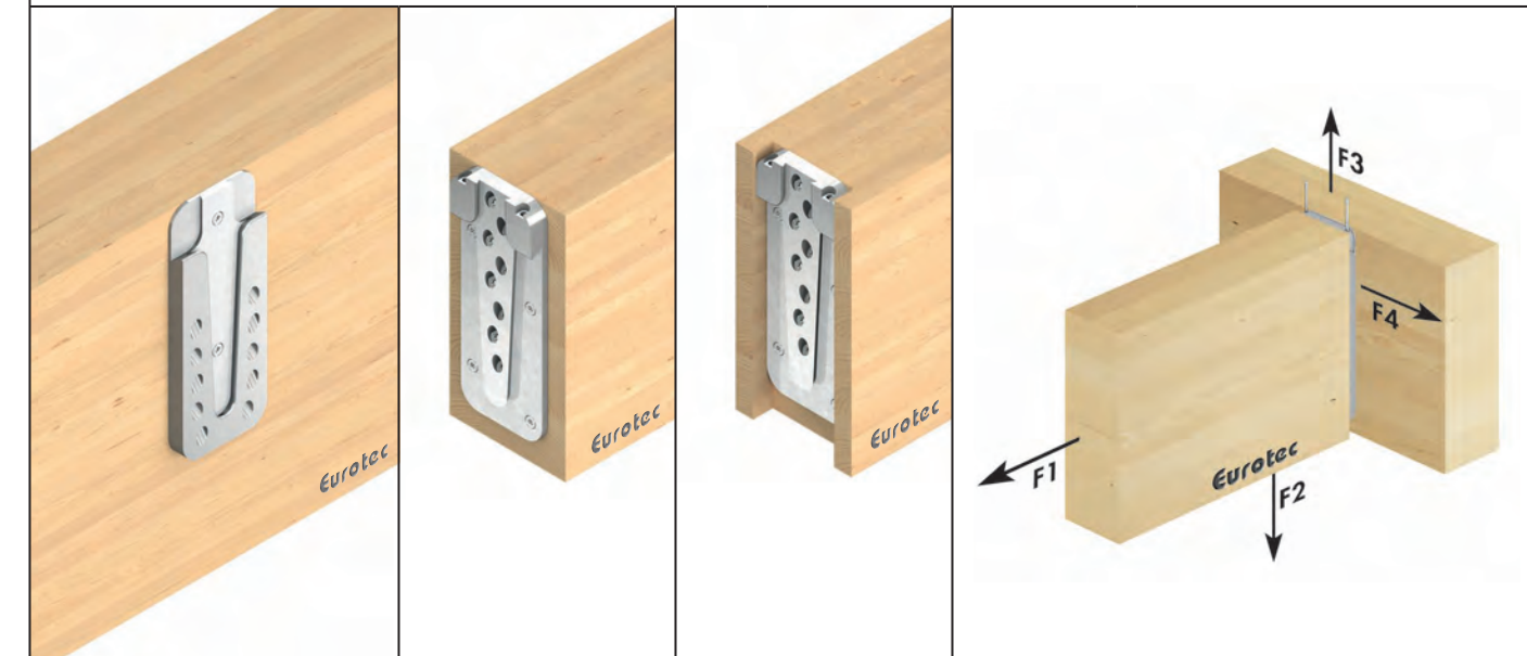
Условные обозначения: пролетная балка, второстепенная балка открытй монтаж, второстепенная балка потайной монтаж, размеры навесок
