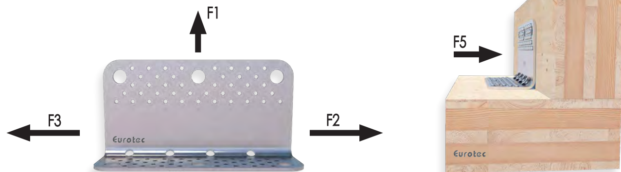
Вектор силы F1Rk; F2/3Rk; F5Rk
